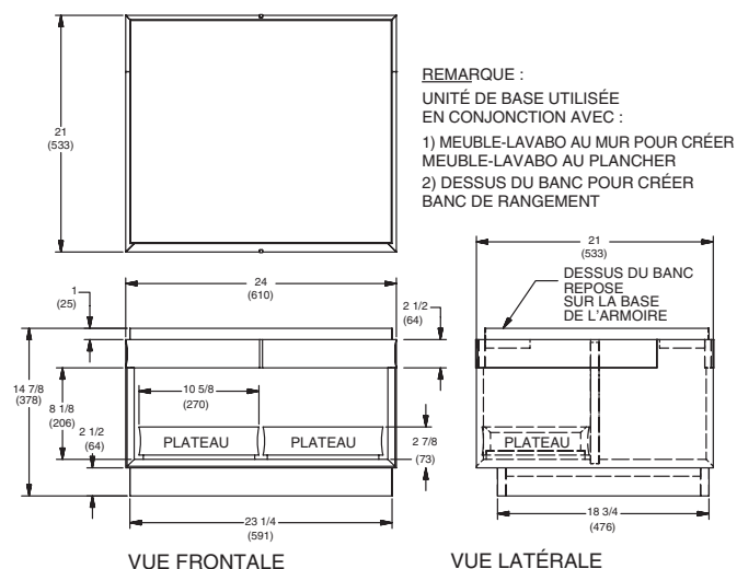
BANC DE RANGEMENT 89120-00
