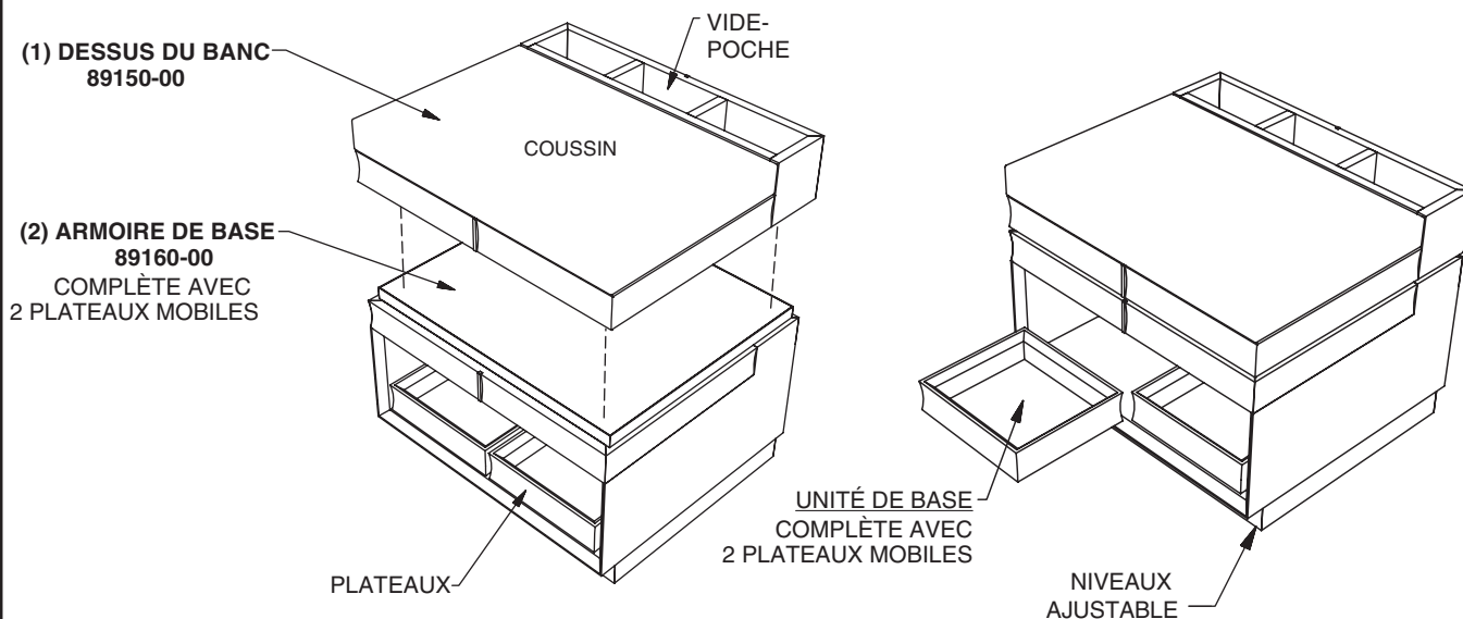
BANC DE RANGEMENT 89120-00
