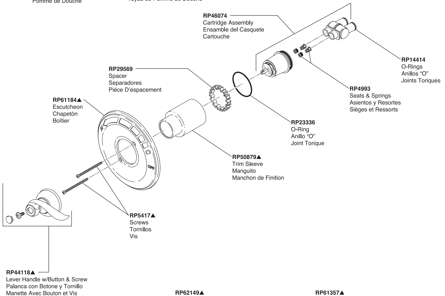
RP62149▲ Tub Spout / Non Diverter Tubo de Salida para Bañera / Sin Desviador Bec / Sans Dérivation
