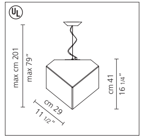
Edge 30 suspension
